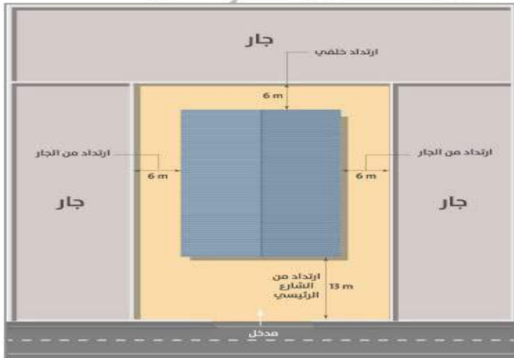
مثال (ب) يوضح الارتدادات في المواقع المعتمدة كمخططات للمصانع
