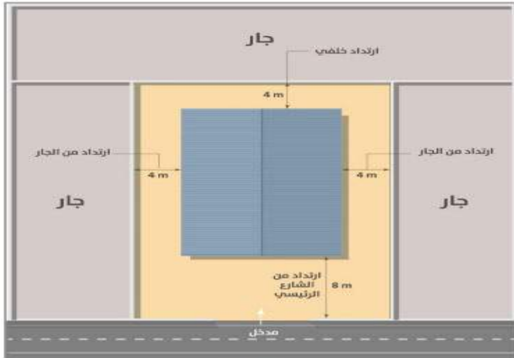
مثال (أ) يوضح الارتدادات لموقع مستقل ومناطق الخدمات المساندة
